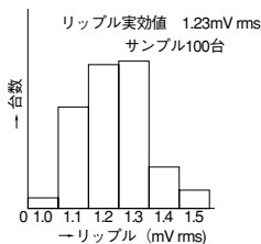
【図-2】リップル (ノイズ)
