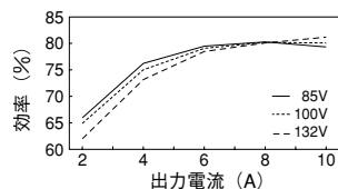
【図-15】 入力電圧別効率の変化
